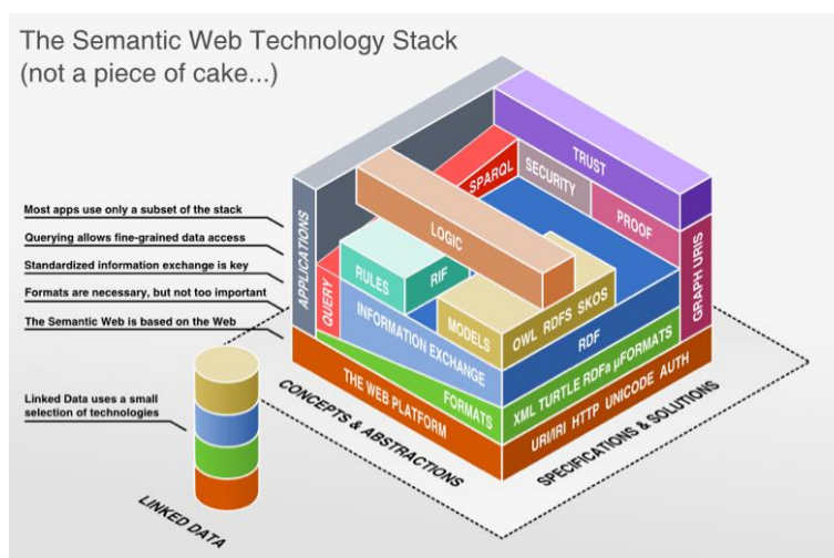
Figura 2. Representación gráfica del conjunto de tecnologías de la Web Semántica (Fuente: http://bnode.org/media/2009/07/08/semantic_web_technology_stack.png )
