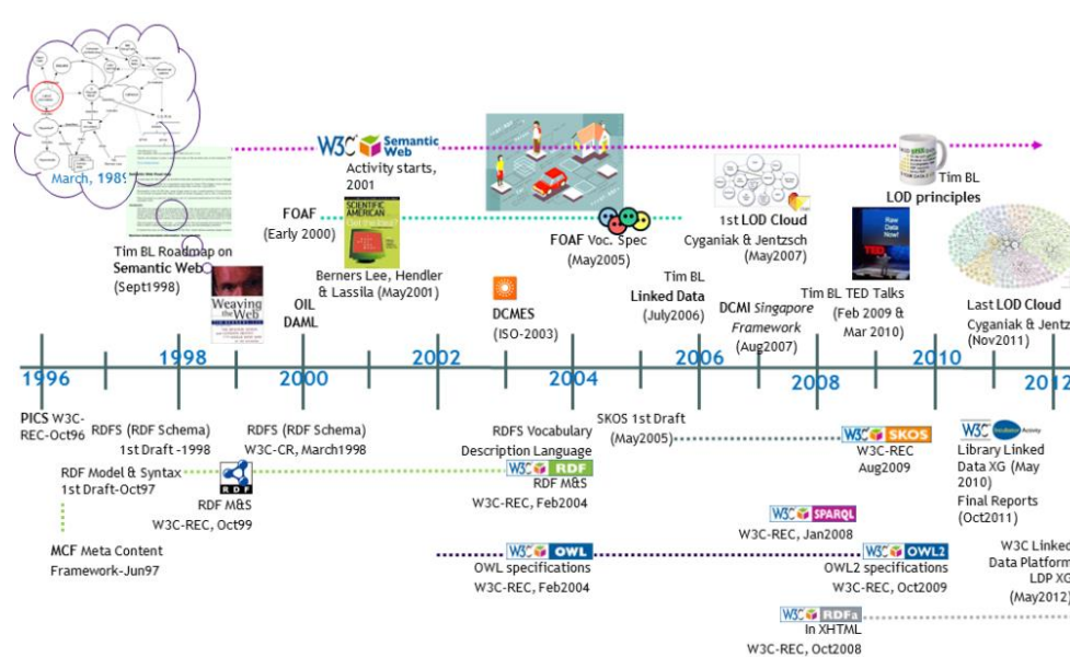
Figura 1. 15 años de web semántica: evolución de los estándares (Mendez, Greenberg, 2012)
